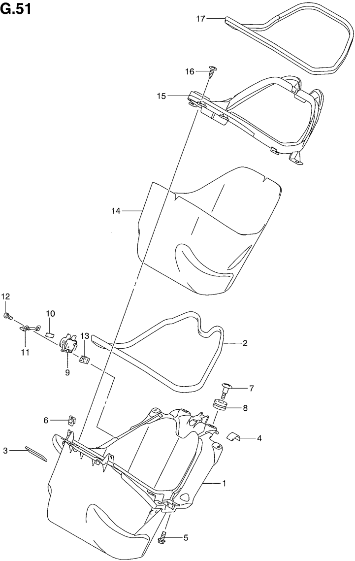
FIG.51 (G-10) ヘルメット ボックス
